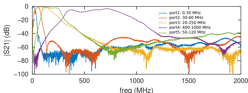
FIGURE 3 – Caractérisation en transmission ( S_{21} ) des filtres passe-bande placés entre chaque connecteur d'antenne et le récepteur radiofréquence MSi001.
