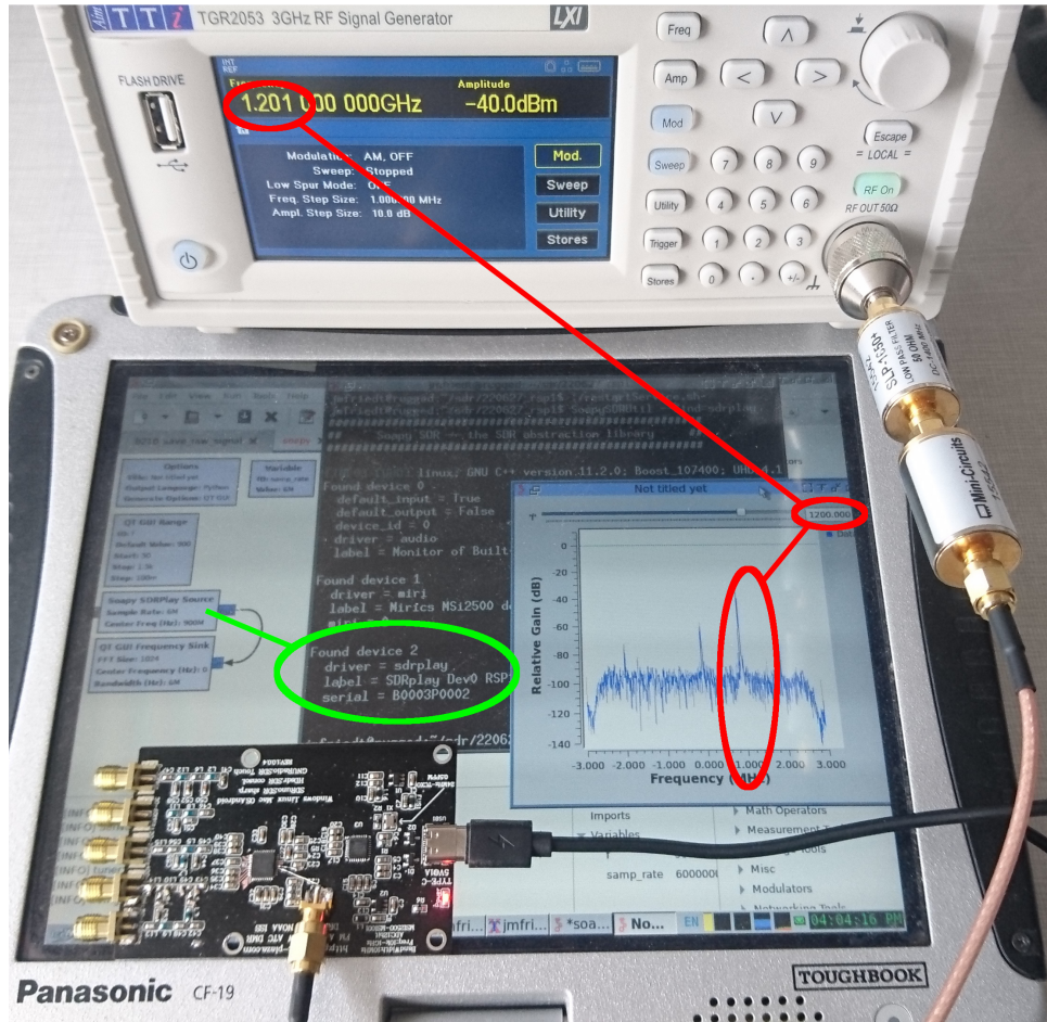
FIGURE 6 – Validation de la capacité du RSP1 modifié par l'ajout du connecteur sur l'entrée de la bande L à recevoir un signal autour de 1200 MHz (ellipses rouges) lorsque réglé sur cette porteuse (ellipses vertes).
