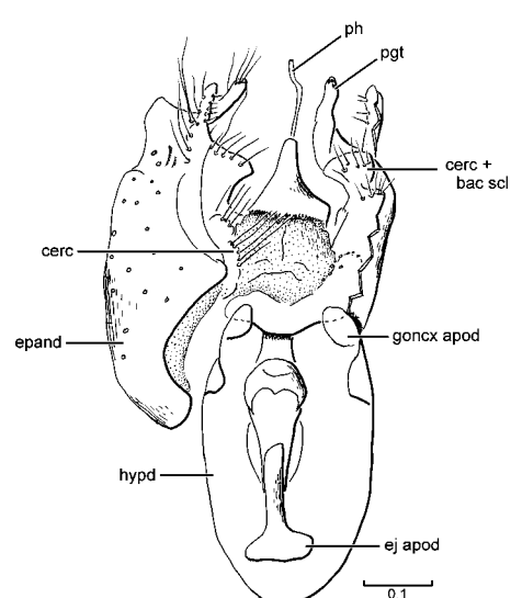
285. Hilara maura
