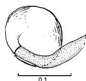
233. Ceratomerus paradoxus
