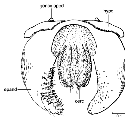
263. Homalocnemis adelensis
