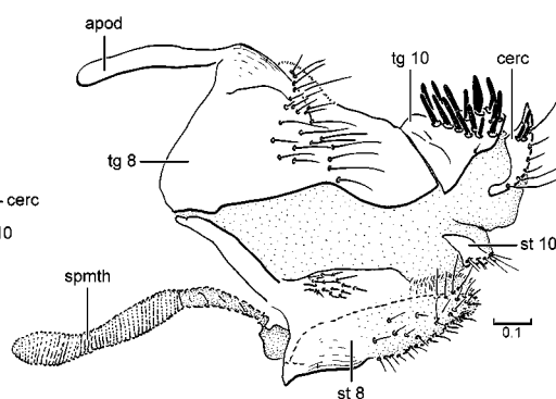
236. Heterophlebus versabilis
