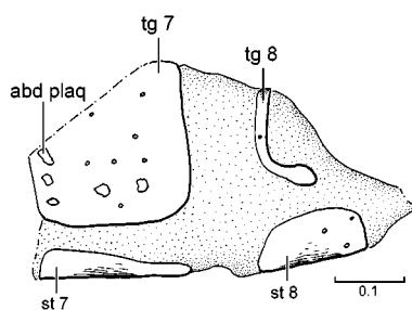
254. Meghyperus sp.
