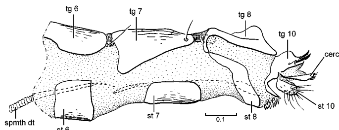
247. Sympycnus anomalipennis
