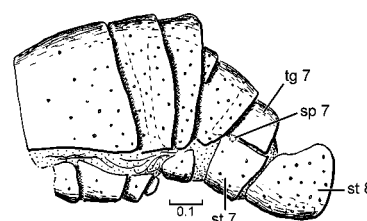
257. Parathalassius aldrichi
