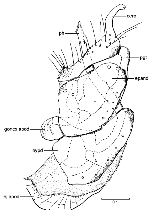
287. Chelipodozus cinereus
