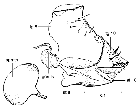
232. Glyphidopeza fluviatilis
