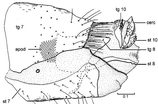
237. Niphogenia eucera
