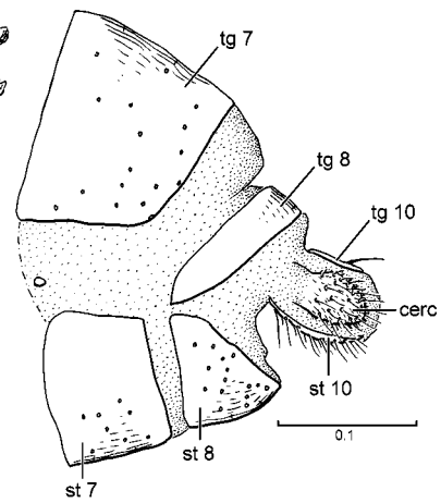
251. Lonchoptera sp.
