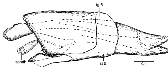
249. Opetia nigra
