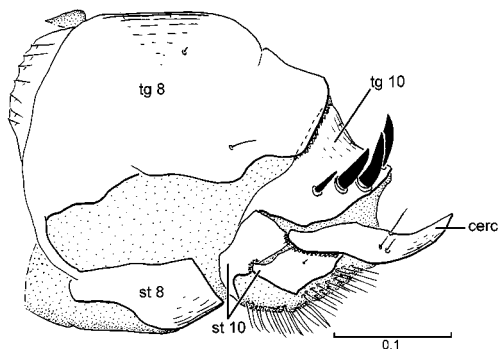
238. Schistostoma armipes
