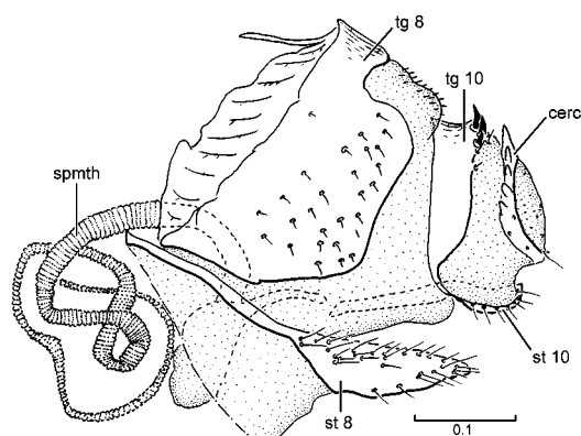
231. Brachystoma nigrimanus
