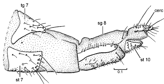
250. Sciadocera rufomaculata
