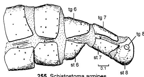
255. Schistostoma armipes
