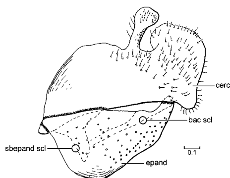
288. Chelifera valida
