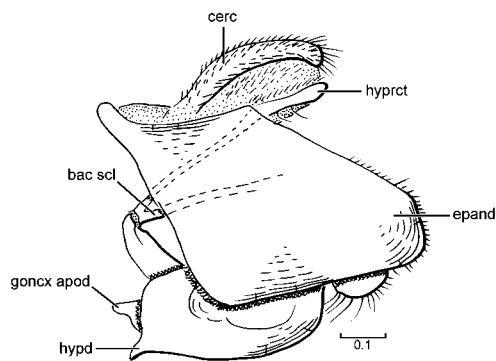
262. Homalocnemis adelensis
