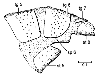
261. Sympycnus anomalipennis
