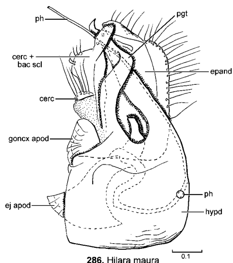
286. Hilara maura
