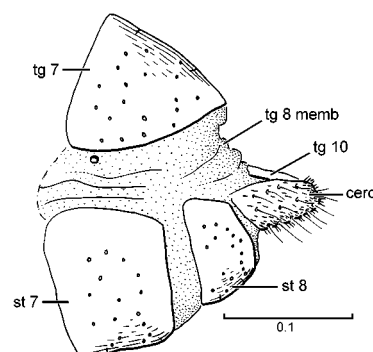
253. Lonchoptera uniseta
