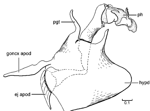
289. Chelifera valida
