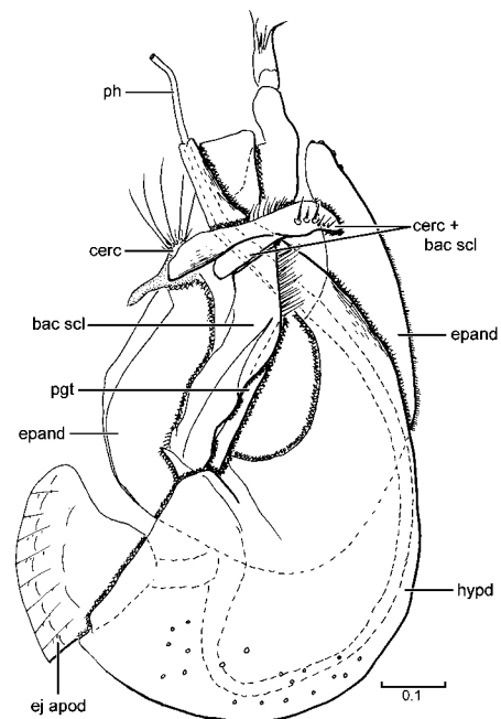
283. Hilarempis facilis
