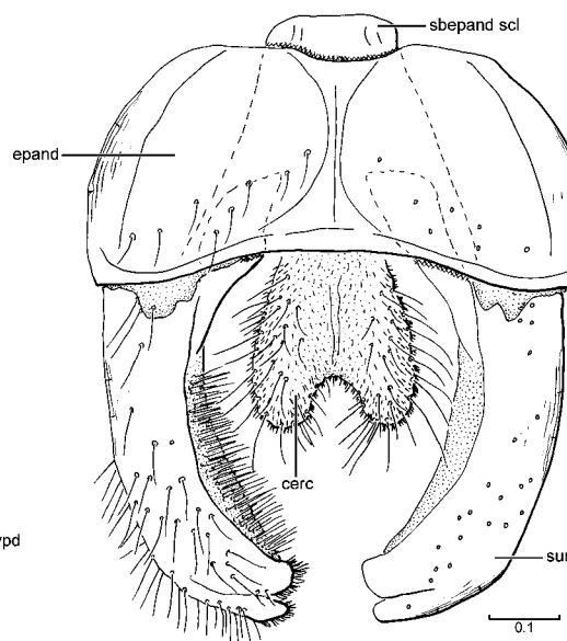
290. Brochella monticola
