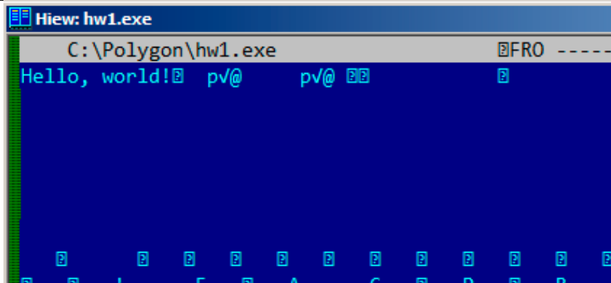
Fig. 5.1: Hiew
