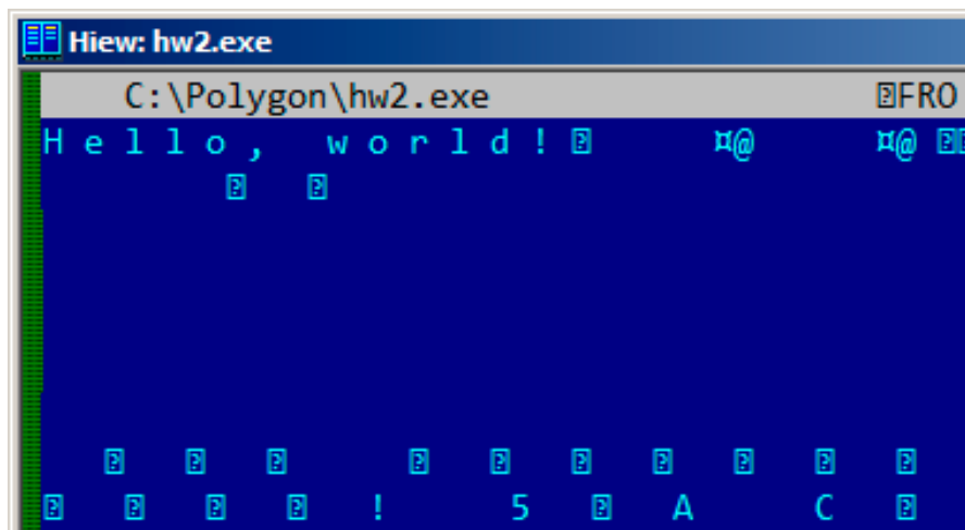
Fig. 5.3: Hiew
