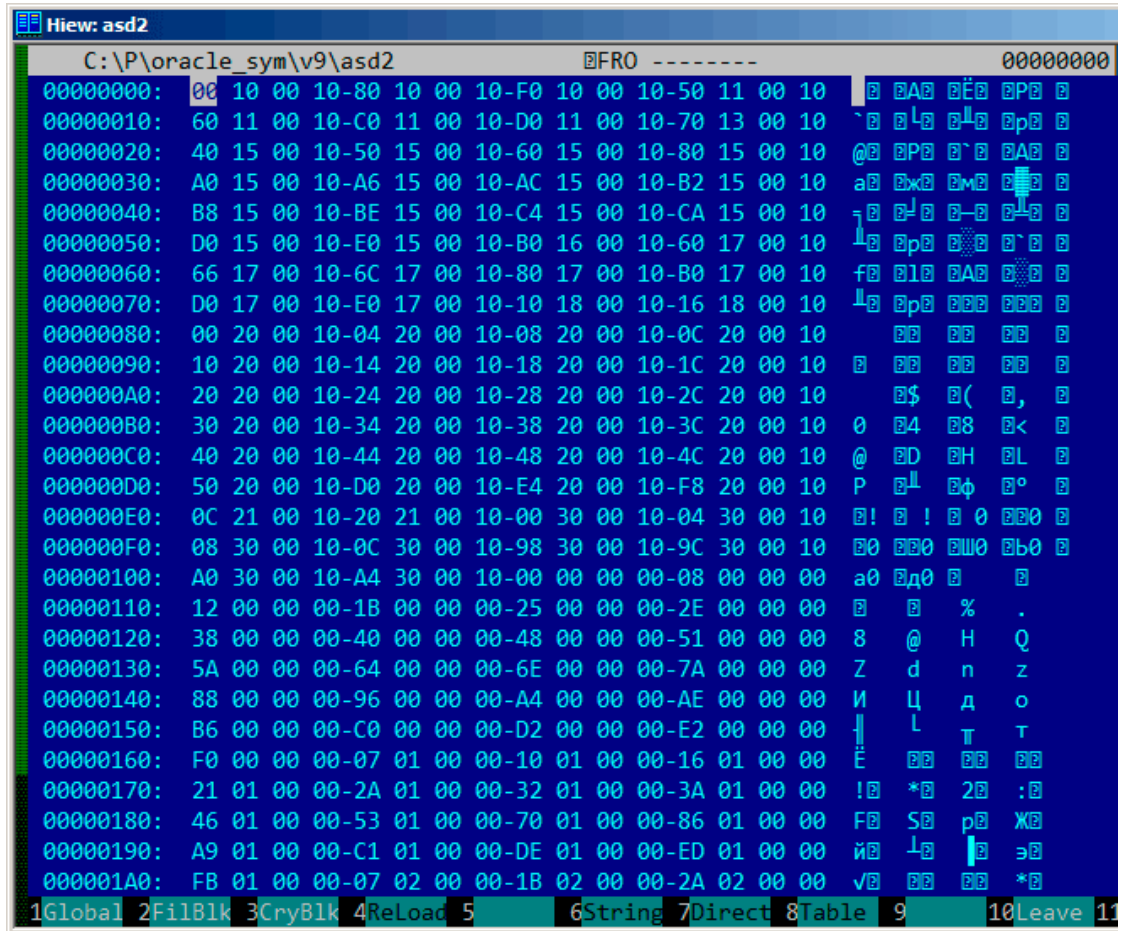
Fig. 9.24: Bloc binaire
