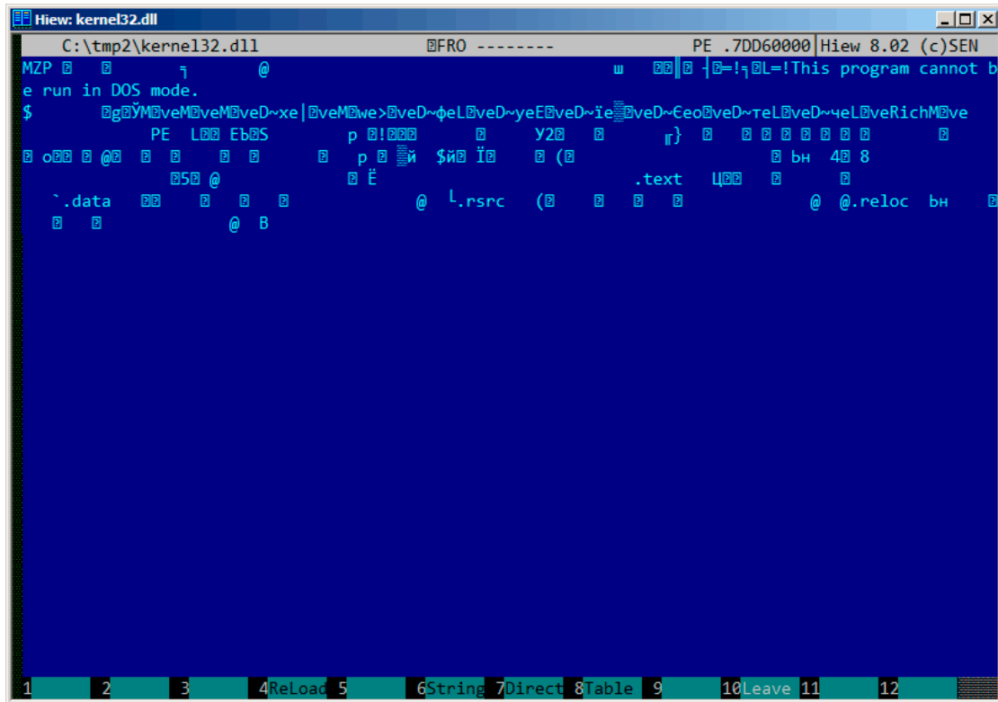
Fig. 9.4: Fichier original
