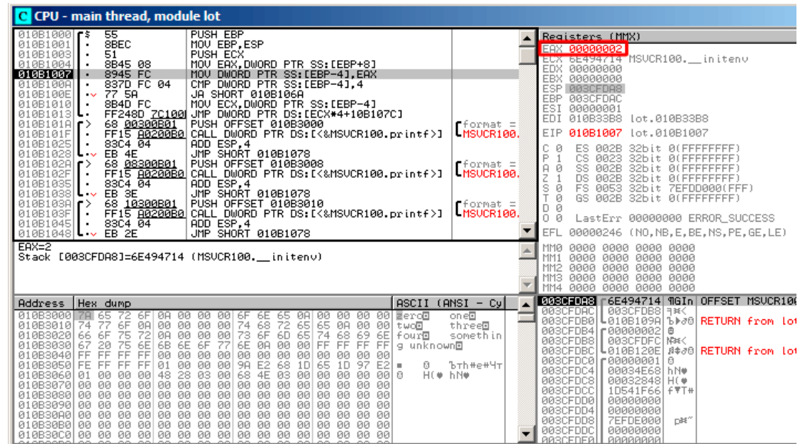
Fig. 1.50: OllyDbg : la valeur d'entrée de la fonction est chargée dans EAX
