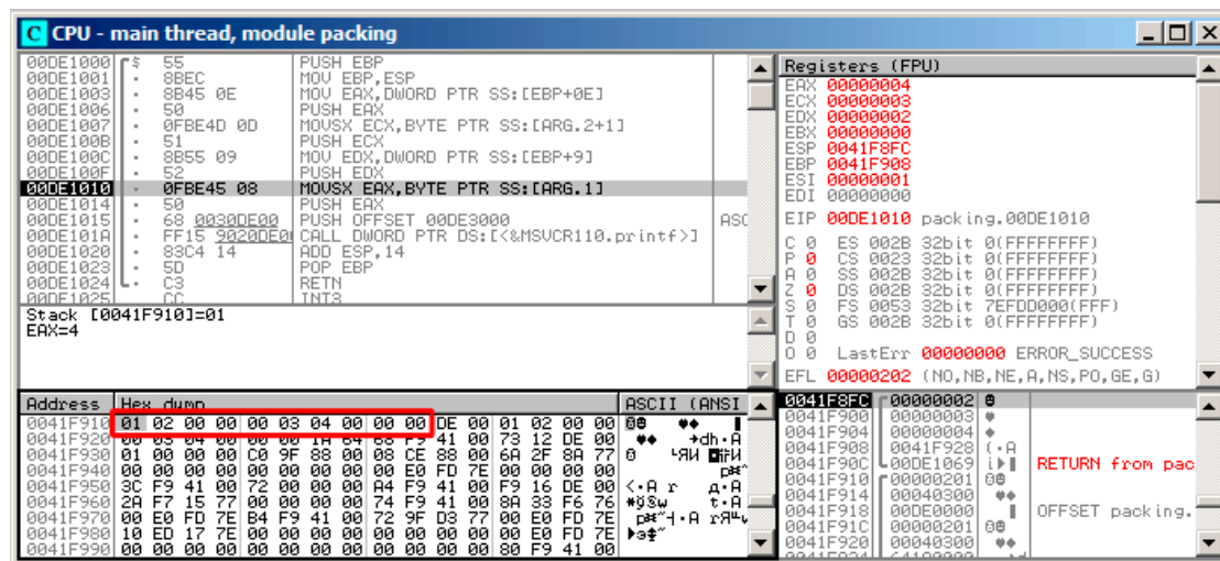
Fig. 1.106: OllyDbg : Avant appel de la fonction printf()
