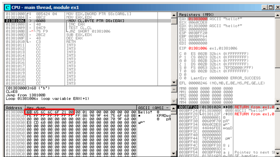
Fig. 1.58: OllyDbg : début de la première itération
