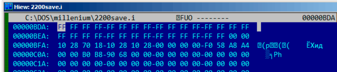
Fig. 9.19: Hiew: mettons les valeurs maximales
