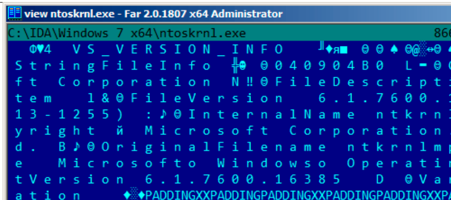
Fig. 5.4: Hiew
