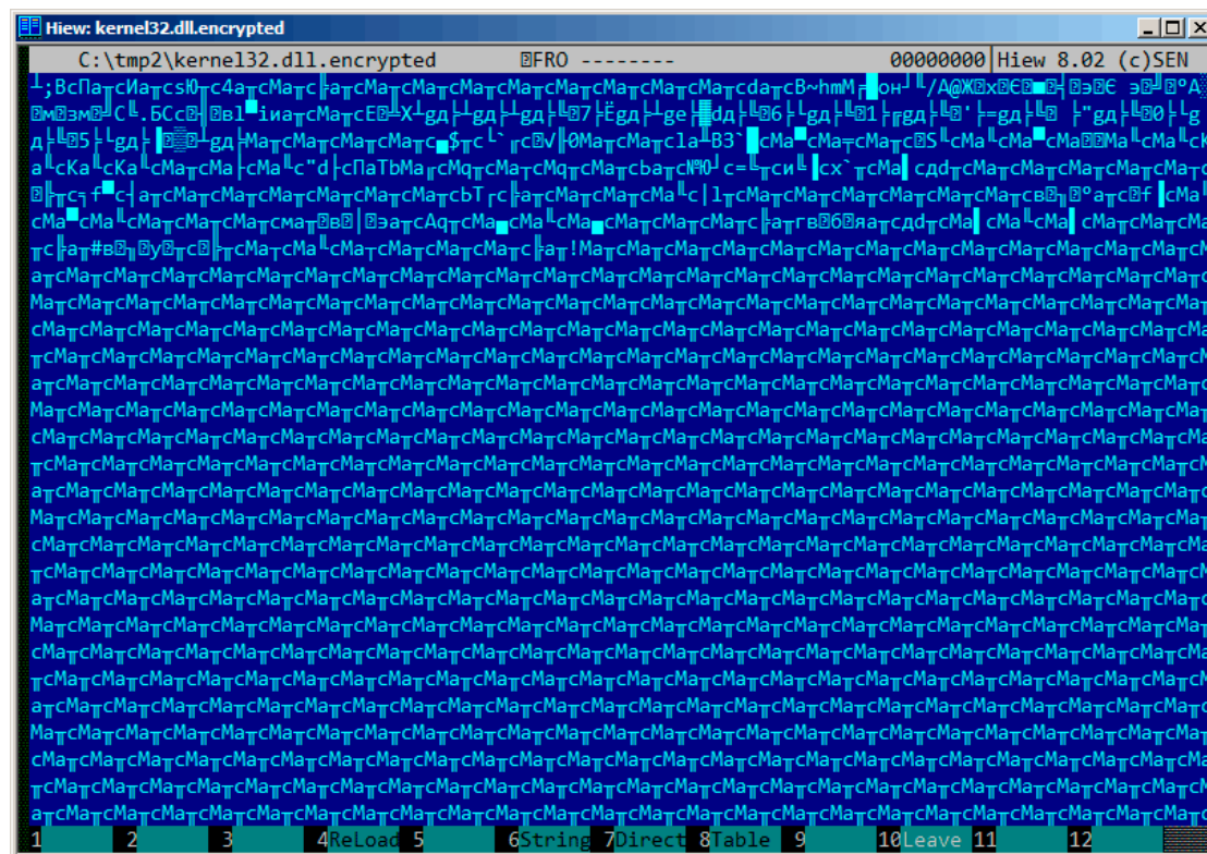
Fig. 9.5: Fichier «chiffré»
