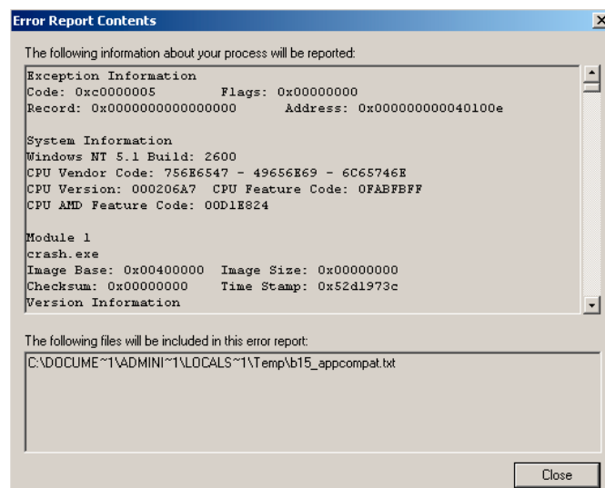
Fig. 6.3: Windows XP
