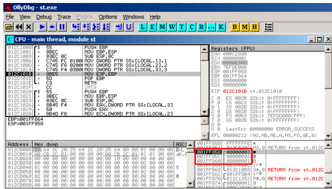
Fig. 1.6: OllyDbg : f1()
