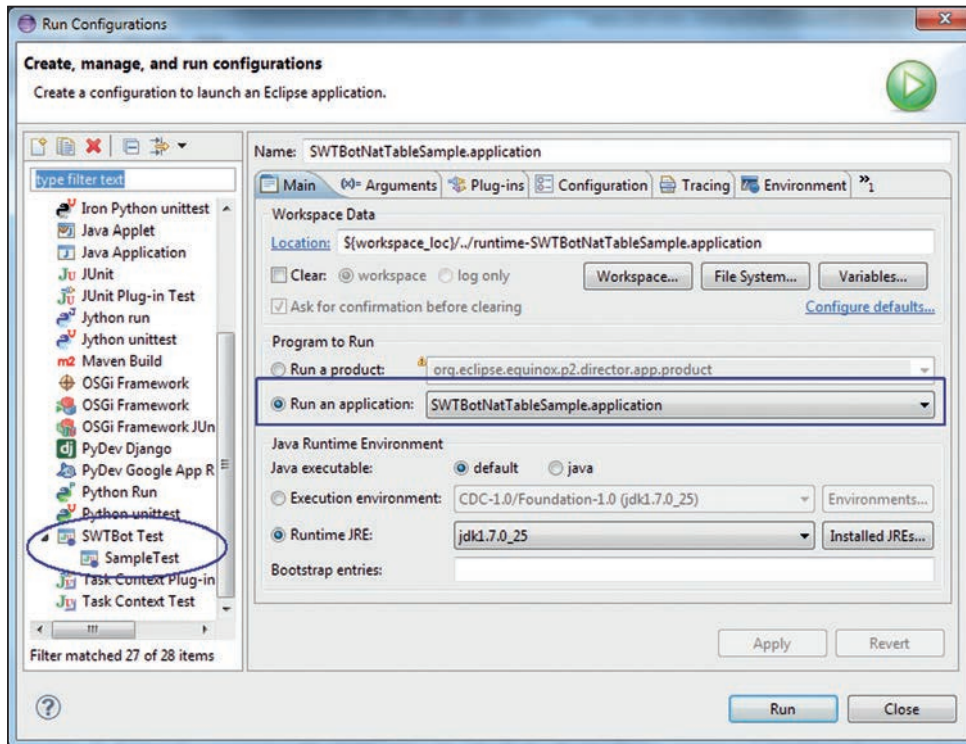
Abb. 2: Anlegen der Run Configuration für den SWTBot-Test in der Eclipse-IDE
