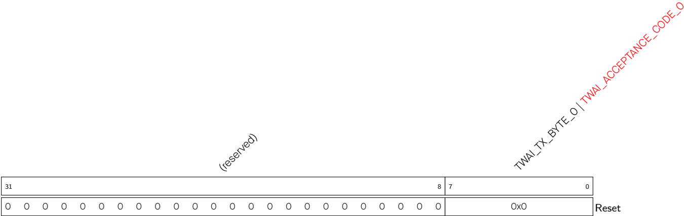
Register 25.5. TWAI_DATA_O_REG (0x0040)
